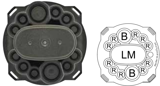
FST 13 Port Base Configuration
