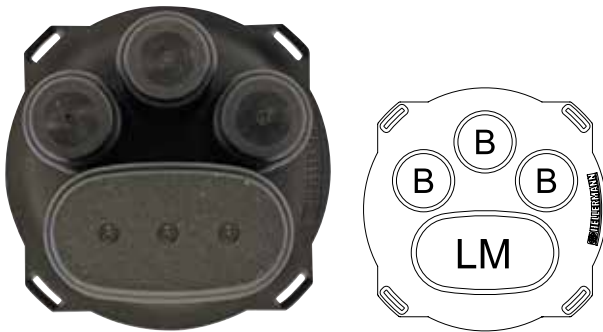
FST 4 Port Base Configuration
