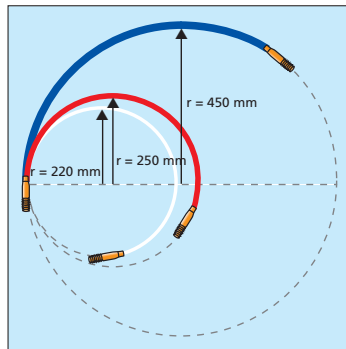
Oversikt over Cable Scout+ marginal bøyeradius
